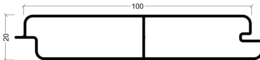
W-25 Lâmina de encaixe 100 x 20
