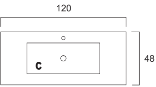
Vista de Frente do Lavatório
