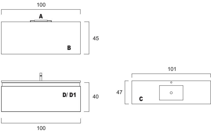
Vista de Cima do Tampo de Vidro
