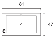
Vista de Cima do Tampo de Vidro
