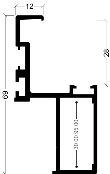
FL-03 Folha semi-estrutural
