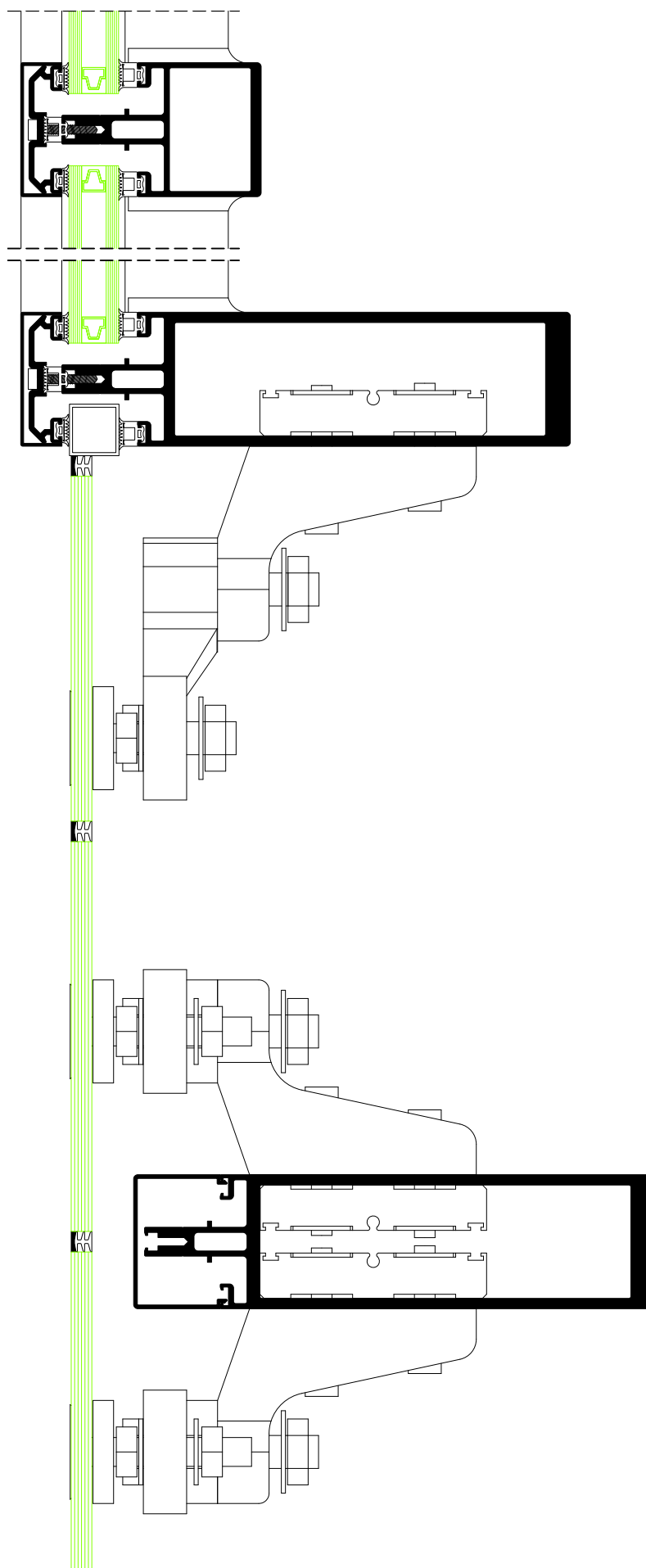
Seção A-A'
