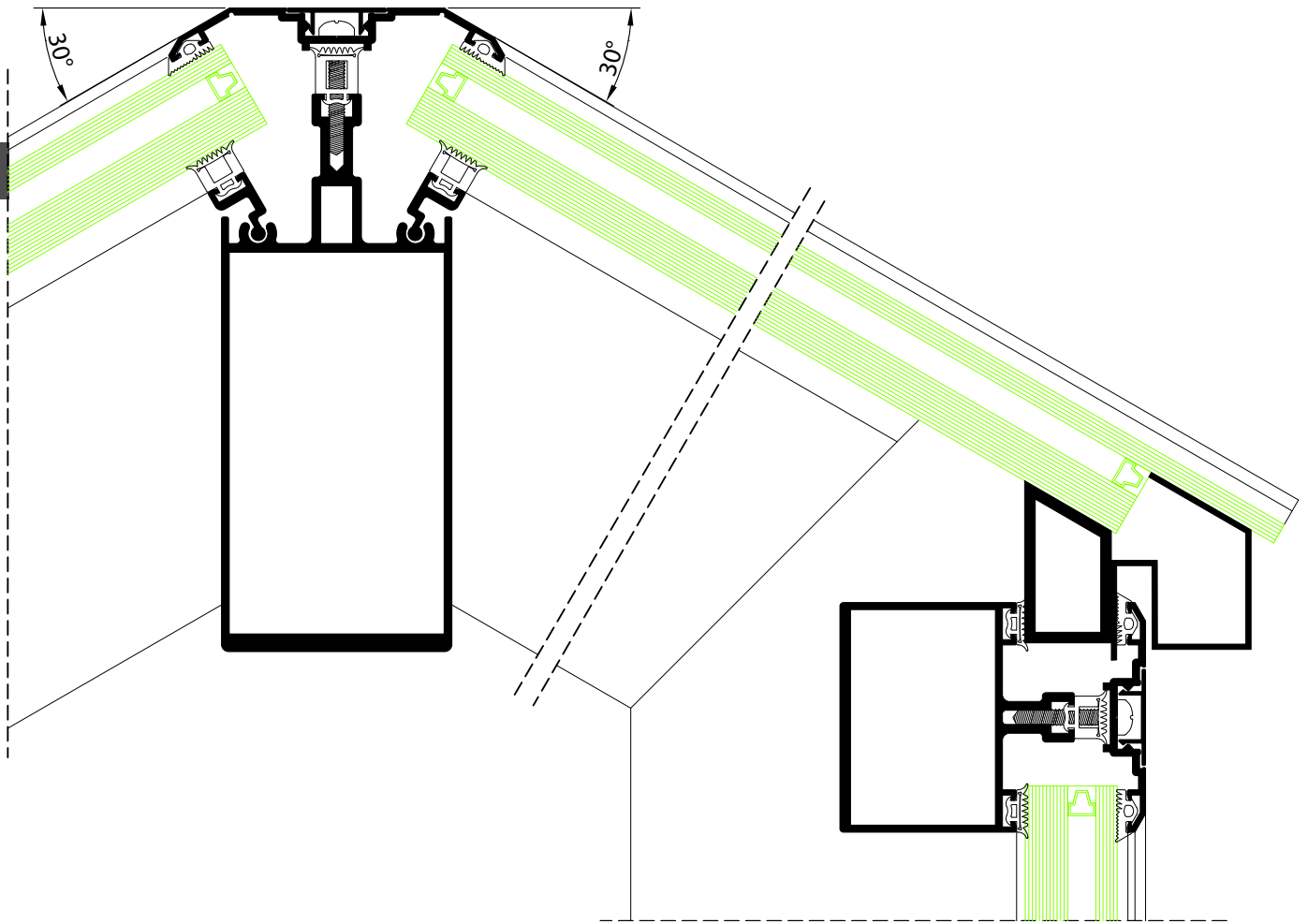
Secção N
