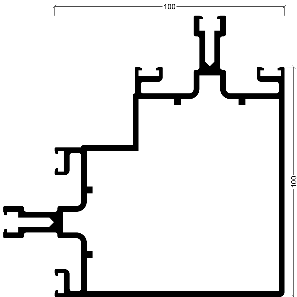
FL-43 Esquina 90°
