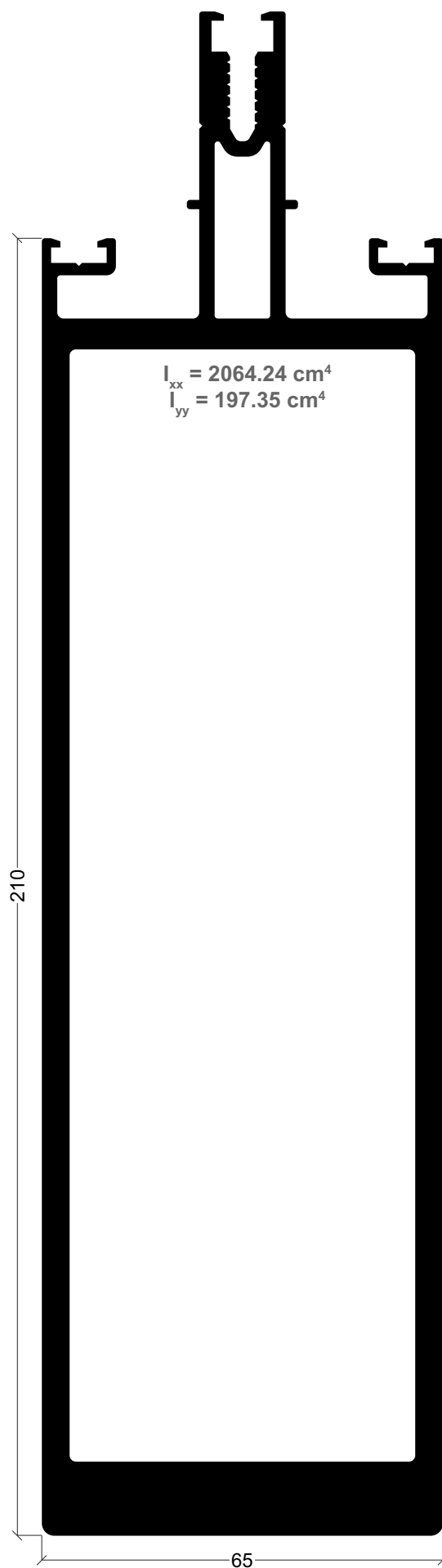
FL-34 Montante de 210 mm
