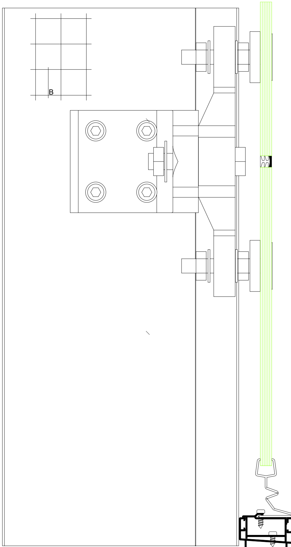
Secção B
