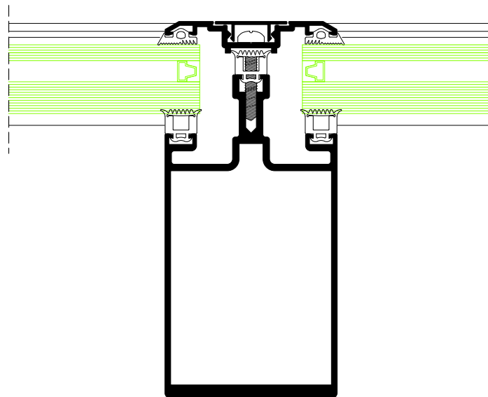
Secção Q
