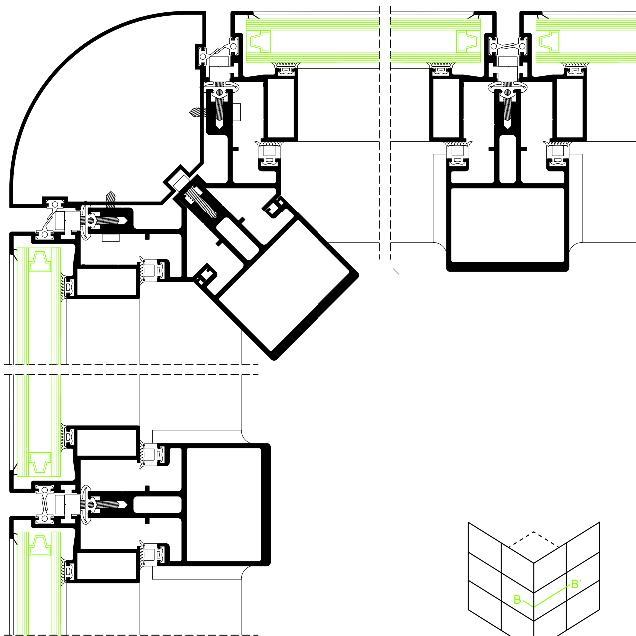
Secção A-A'
