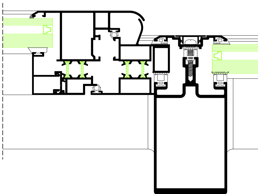
Secção M
