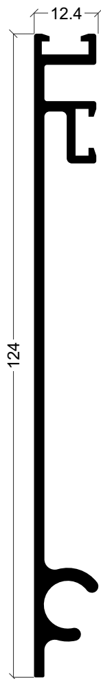
FL-62 Suporte montante basculante
