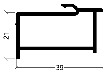
FL-55 Porta-vedante
