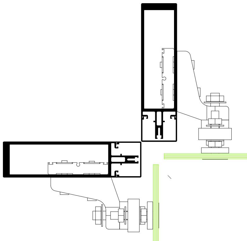
Secção B-B'
