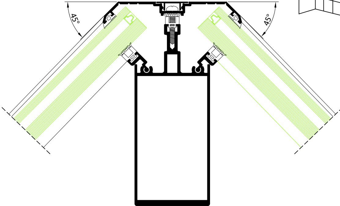
Secção P
