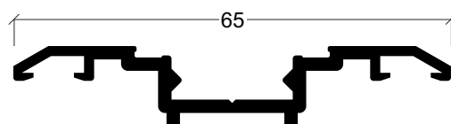
FL-44 Contra tampa
