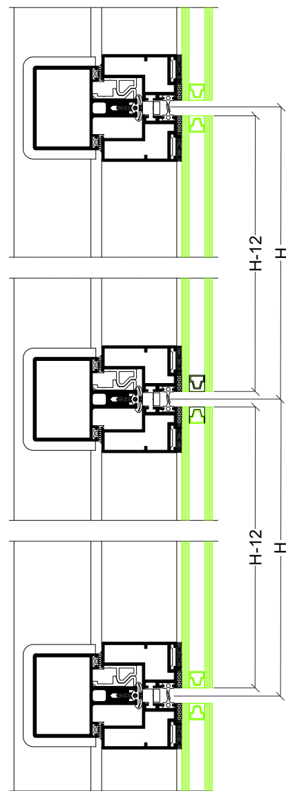
Seção A-A
