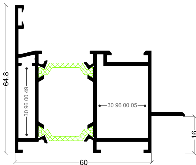
ARi-68 Aro fixo para apanelado
