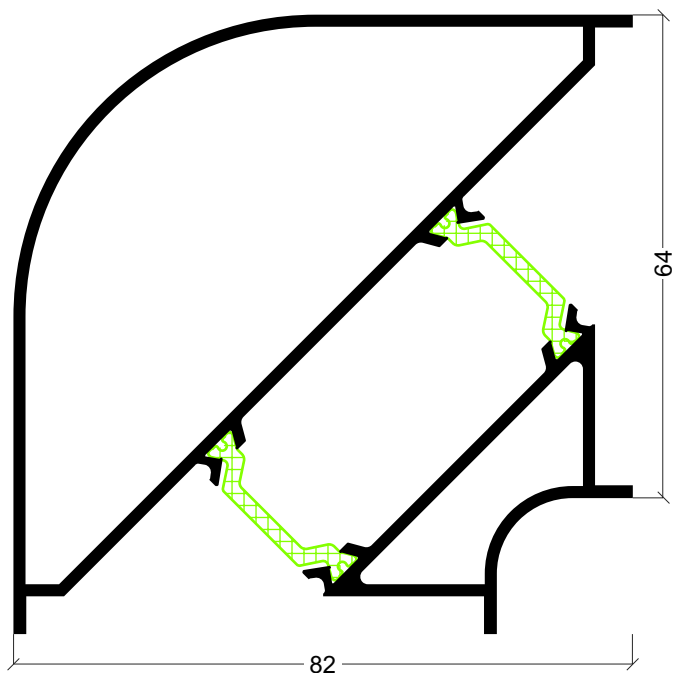
ARi-16 Esquina 90°
