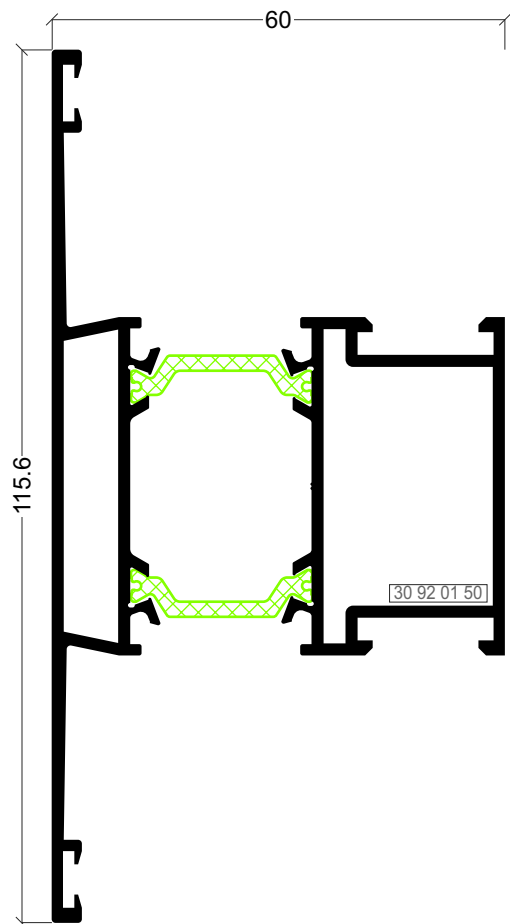
ARi-70 Travessa
