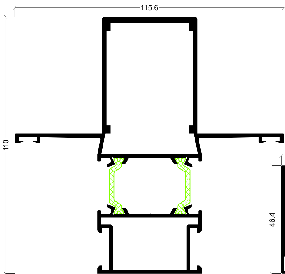
ARi-54 Montante
