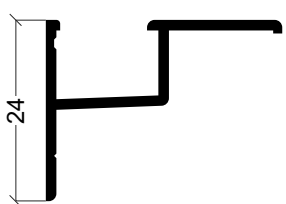
Y-20 Recolha de águas condensação
