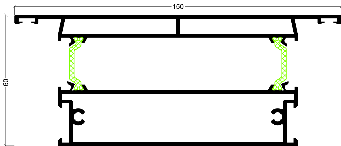
ARi-13 Traversa
