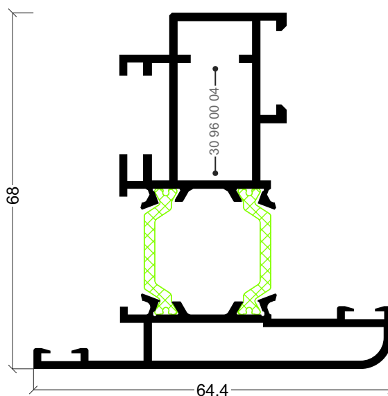
ARI-02 Aro móvel pivotante
