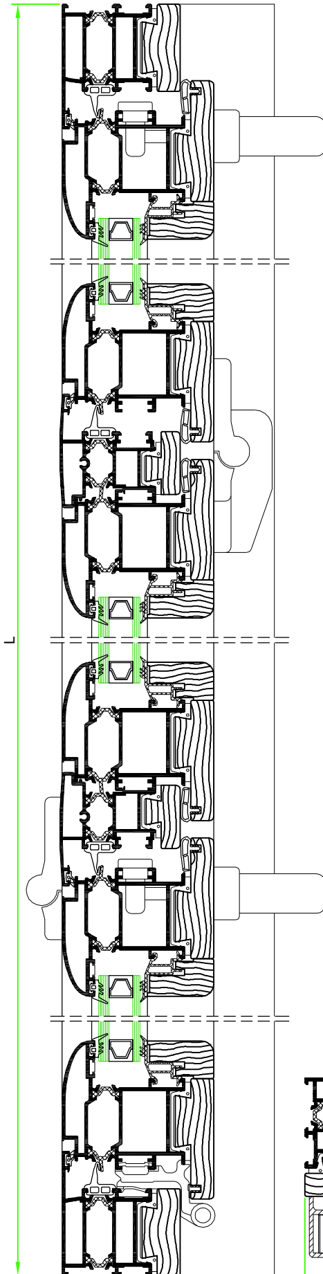
SECÇÃO A - A
