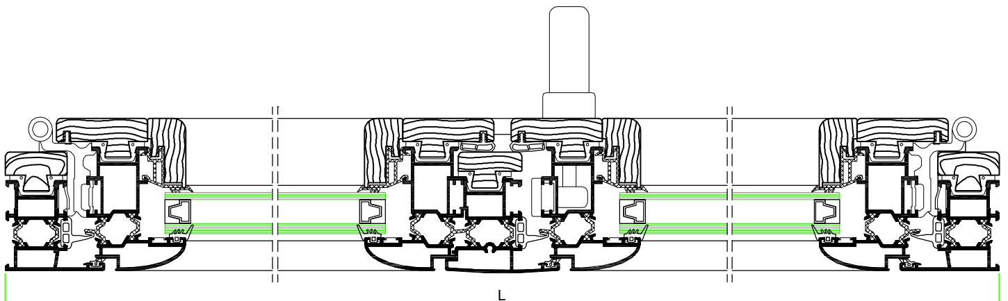
SECÇÃO A - A
