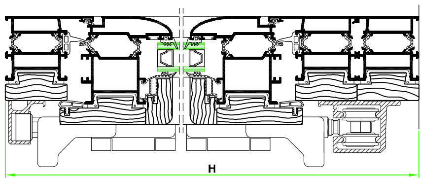
SECÇÃO B - B
