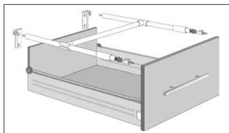
Laterais de gaveta Integra Art. Nr. F084 07. ...
