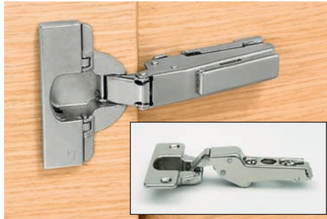
Dobradiça NEXIS Click-on - Ângulo de 100° Art. Nr. F015 072 ...
