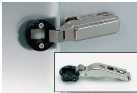
Dobradiça NEXIS Click-on para portas de vidro Ângulo de 94° Art. Nr. F015 072 80.
