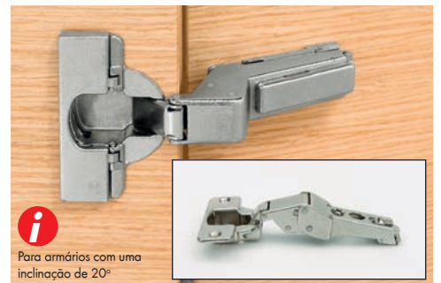
Dobradiça NEXIS Click-on - Ângulo de 94° Art. Nr. F015 072 684
