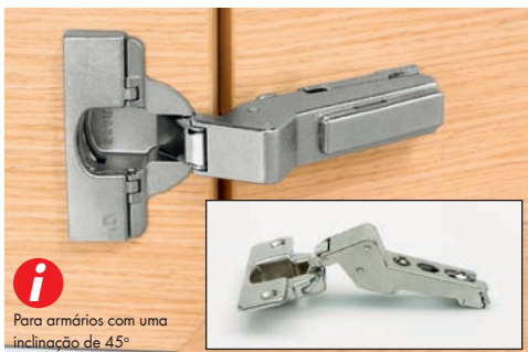
Dobradiça NEXIS Click-on - Ângulo de 94° Art. Nr. F015 072 67.
